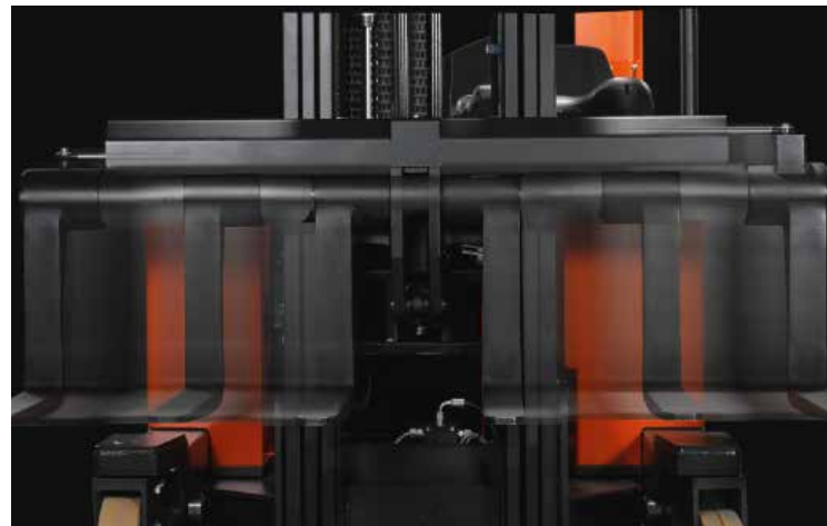
BT Reflex F-sarjan asetinlaitteen haarukoiden leveyden säätö helpottaa eripituisten kuormien turvallisen käsittelyn
